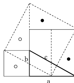
図16 問題例②
