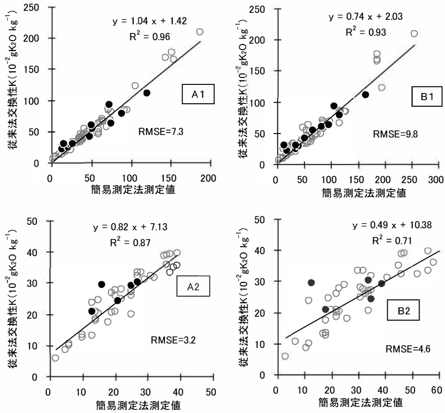
第4-1図 簡易測定法での測定値(減法値)と従来法での交換性Kとの関係
