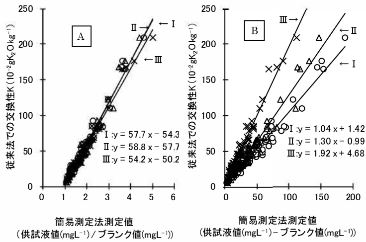
第4-2図 測定ベースラインの水準が異なる条件における高 AAs 抽出測定での測定値計算法が従来法交換性K との関係に及ぼす影響
