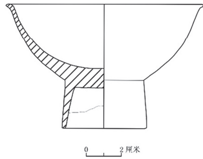
图四, 3 宋代青白釉高足盞 圆唇微外卷, 敞口, 鼓腹, 高圈足, 釉色呈青绿色, 唯足底露胎, 应为湖田窑烧造。
