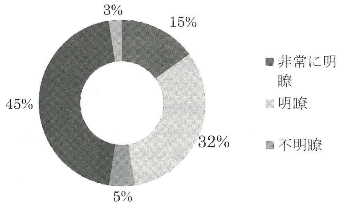
図一六 地震によって発生した斜面崩壊箇所の遷急線の有無の割合 (n=40)
