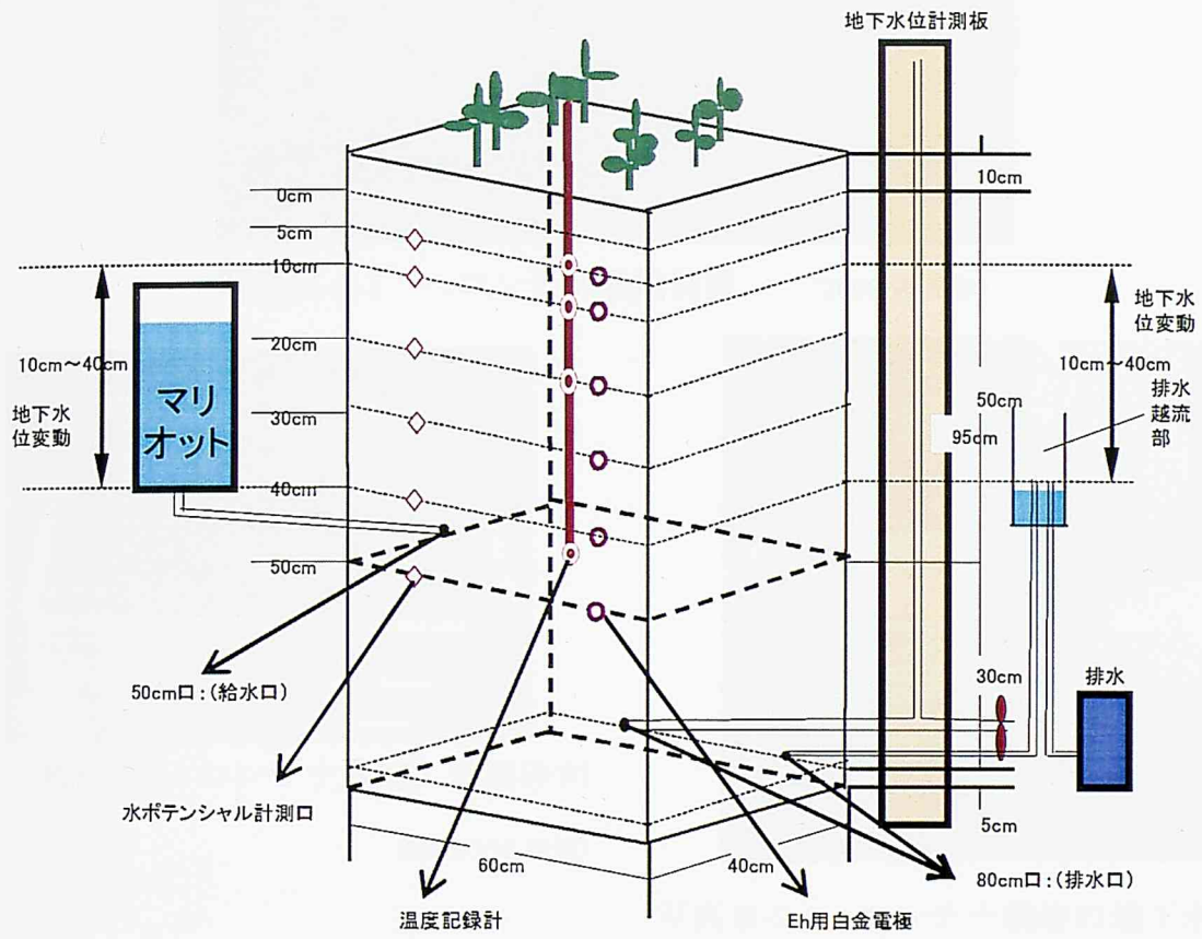
図III-2-1 コンテナ栽培装置の概要
