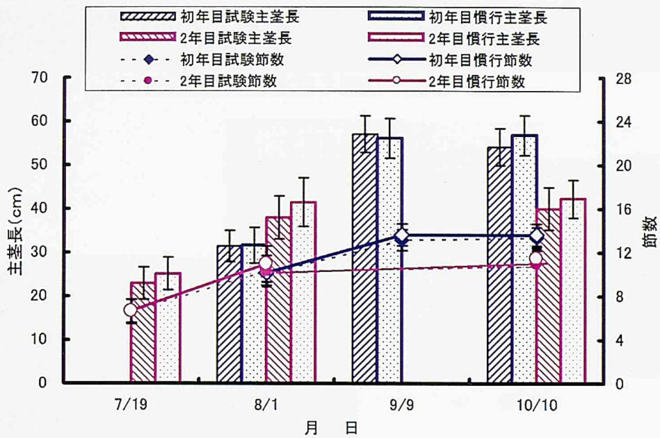
図 II -3-5 試験区と慣行区の生育状況（主茎長および節数）
