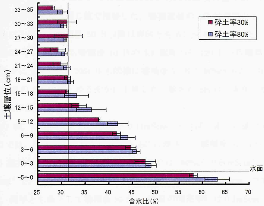
図III-3-5 砕土率 80%土壌と砕土率 30%土壌の毛管上昇
