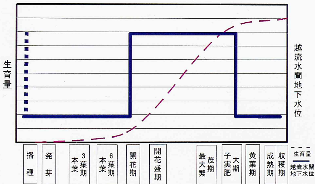
図 I-3 多収ダイズのための地下水位制御の考え方
