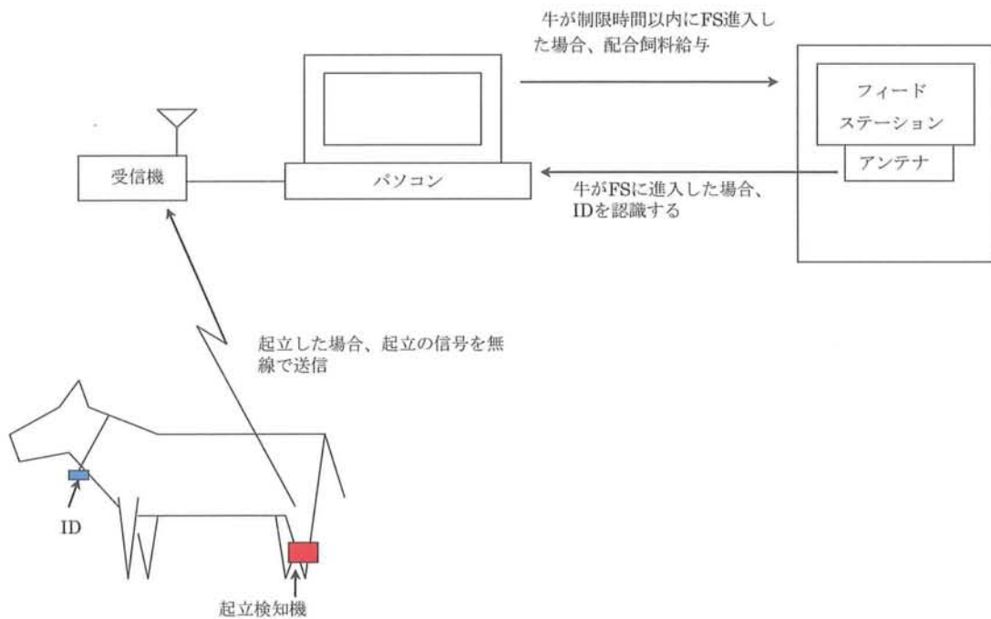
図 4. 起立検知ならびに FS 制御システム
