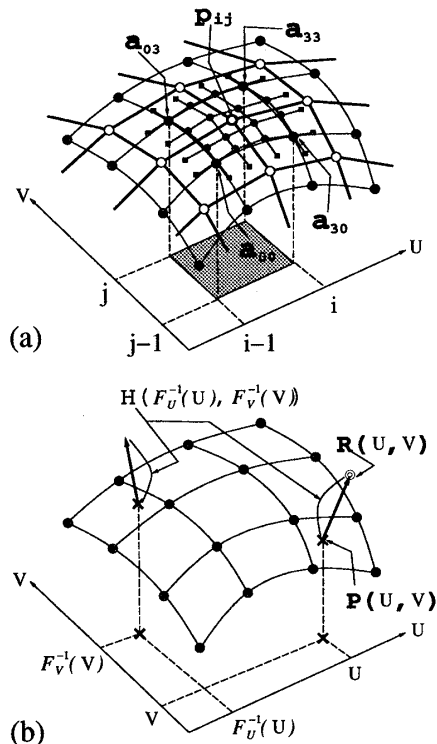
図2 正方メッシュ上の wrinkly 曲面: (a) 白丸は wrinkly 制御点, 黒丸は Bézier 制御点 (大黒丸は 4 隅の制御点), 黒四角は \mathbf{p}_{ij} に対する Bézier パッチに隣接する周囲の Bézier パッチの制御点の一部を表す. (b) パラメータ (U, V) に対して, 基準曲面上の点 \mathbf{P}(U, V) から法線方向に高さ H(\mathcal{F}_U^{-1}(U), \mathcal{F}_V^{-1}(V)) だけ持ち上げた点を wrinkly 曲面上の点 \mathbf{R}(U, V) とする.
