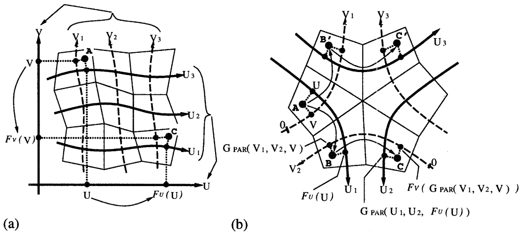
(a) 正方メッシュの場合. U_1, U_2, U_3 軸は U 軸, V_1, V_2, V_3 軸は V 軸によって, それぞれ原点と方向を一致させて代表させることが可能であり, U, V の 2 軸のみに独立に IST を適用するだけでよい. (b) 不規則メッシュの場合. 「 U \rightarrow V 」順序でのグローバル値の変換は A((U_1, U), (V_1, V)) \xrightarrow{U \text{ 方向}} B((U_1, \mathcal{F}_U(U)), (V_2, G_{PAR}(V_1, V_2, V))) \xrightarrow{V \text{ 方向}} C((U_2, G_{PAR}(U_1, U_2, \mathcal{F}_U(U))), (V_2, \mathcal{F}_V(G_{PAR}(V_1, V_2, V)))) となる. ここで関数 G_{PAR} は 3.2.3 項で述べた平行なグローバル軸間でのグローバル値の変換を行う関数である (ここでは G_{PAR} に引数として与える各軸の番号を U_1, U_2, V_1, V_2 のように記述した). たとえば, 図中の点 A, B は各々グローバル軸 V_1, V_2 上で V 値を与えられるが, V_1 と V_2 では原点および軸方向が異なるため, それぞれの V 値は同じ値にはならない. よって, A \xrightarrow{U \text{ 方向}} B の変換時には, グローバル軸 U_1 に沿って反復交差変換 \mathcal{F}_U により U 値を変換すると同時に, V 値に関しても G_{PAR} によって変換を行わなければならない.
