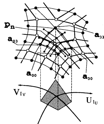
図 9 不規則メッシュ上の wrinkly 曲面: 白丸は wrinkly 制御点, 黒丸は Bézier 制御点 (大黒丸は 4 隅の制御点), 黒四角は p_n に対する Bézier パッチに隣接する周囲の Bézier パッチの制御点の一部を表す. ハッチングされた四角領域は p_n に割り当てられたパラメータ領域, U_{Iu}, V_{Iv} はグローバル軸である.
