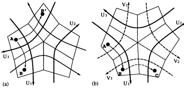
図5 2次元反復交差変換の妥当性：(a) 1系統の例。2段階の変換を行う場合、仮に U_1 軸方向を1回目の変換方向として選択すると、 U_1 軸に平行な U_2 軸、そして、 U_2 軸に平行な U_3 軸も1回目として同時に選択される。その結果、 U_1, U_3 軸を持つパッチ上の点 A はどちらの軸方向に1回目の変換を行うべきか(点 B と B' のいずれか)決定できなくなる。(b) 2系統の例。同系統に属する2軸を持つパッチが存在しないため、(a)のような不都合が生じない( A \xrightarrow{U \text{ 軸方向}} B \xrightarrow{V \text{ 軸方向}} C )。
