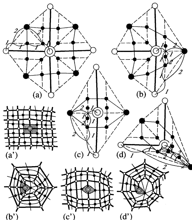
図 10 Bézier パッチの制御点の計算：白丸は wrinkly 制御点、黒丸は Bézier パッチの制御点を表す。(a), (b), (c) および (d) は中央の wrinkly 制御点 (二重白丸) に対する Bézier 制御点の計算方法、(a'), (b'), (c') および (d') はその各々が実際のメッシュ中で現れる例 (色の付いた部分が対象となる Bézier パッチ) を示す。(b), (c), (d) の Bézier パッチは縮退し、いくつかの Bézier 制御点が重なることで、3 辺形、2 辺形となる。
