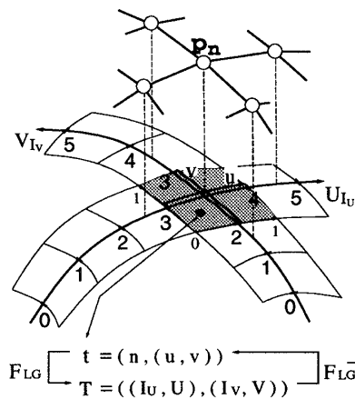
図6 ローカル軸のグローバル軸への埋め込み：白丸は wrinkly 制御点を表す。 U_{I_U}, V_{I_V} はそれぞれ軸番号 I_U, I_V のグローバル U, V 軸である。色付きの四角領域は wrinkly 制御点 p_n に割り当てられたパラメータ領域(領域内の矢印線でローカル u, v 軸を表す)であり、その内部の点はローカル座標値 t およびグローバル座標値 T で特定化される。
