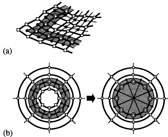
図 11 境界を持つ制御メッシュ：白丸は wrinkly 制御点，二重白丸は境界上の wrinkly 制御点，白四角は仮の wrinkly 制御点，黒丸は Bézier パッチの 4 隅の制御点を表す。(a) 仮の wrinkly 制御点は境界上の Bézier パッチ（色付き）を定義するために配置される。(b) 仮の wrinkly 制御点を取り去ることで中央の境界が閉じる。中央の Bézier パッチ（色付き）が 3 辺形に縮退する。
