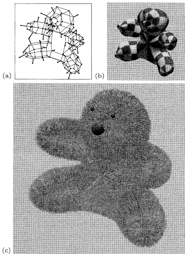
図 14 Wrinkly 曲面を用いた形状モデルの例：(a) 制御メッシュ（格子点上に wrinkly 制御点が位置し、先の丸いトゲで高さ値分の法線方向への持ち上げを表す）。(b) 各 wrinkly 制御点に対する 3 次 Bézier パッチ。隣接するパッチを互いに色分けして示している。IST は適用せず高さ H(t) 分をそのまま法線方向に持ち上げて表示した。(c) wrinkly 曲面（色は 1 色とし、鼻と目は別データとして付加）。
